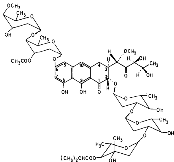
Fig. 1. Olivomycin.
